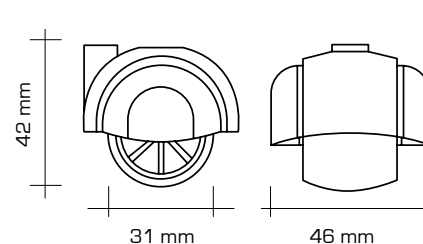
LEM UNO Ø40
